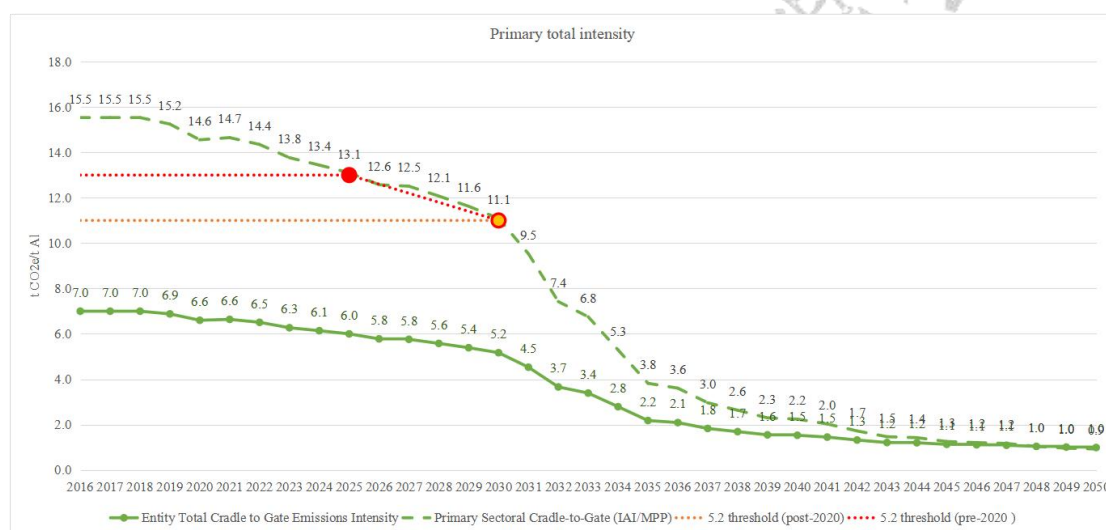
图 1 云铝海鑫从矿山到金属铝铸锭的排放强度 1.5°C减排目标
